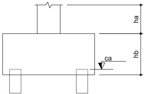
2 BLOCOS DE FUNDAÇÃO ESCALA: 1/25
