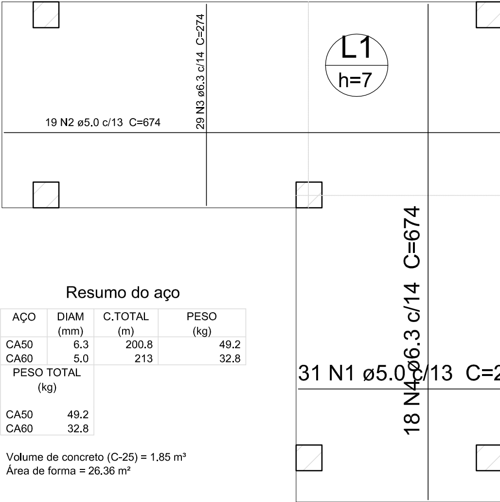
5 LAJE NÍVEL 000 SEM ESCALA
