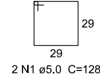
4 PILARES NÍVEL 000 E BL. DE FUNDAÇÃO ESCALA: INDICADA
