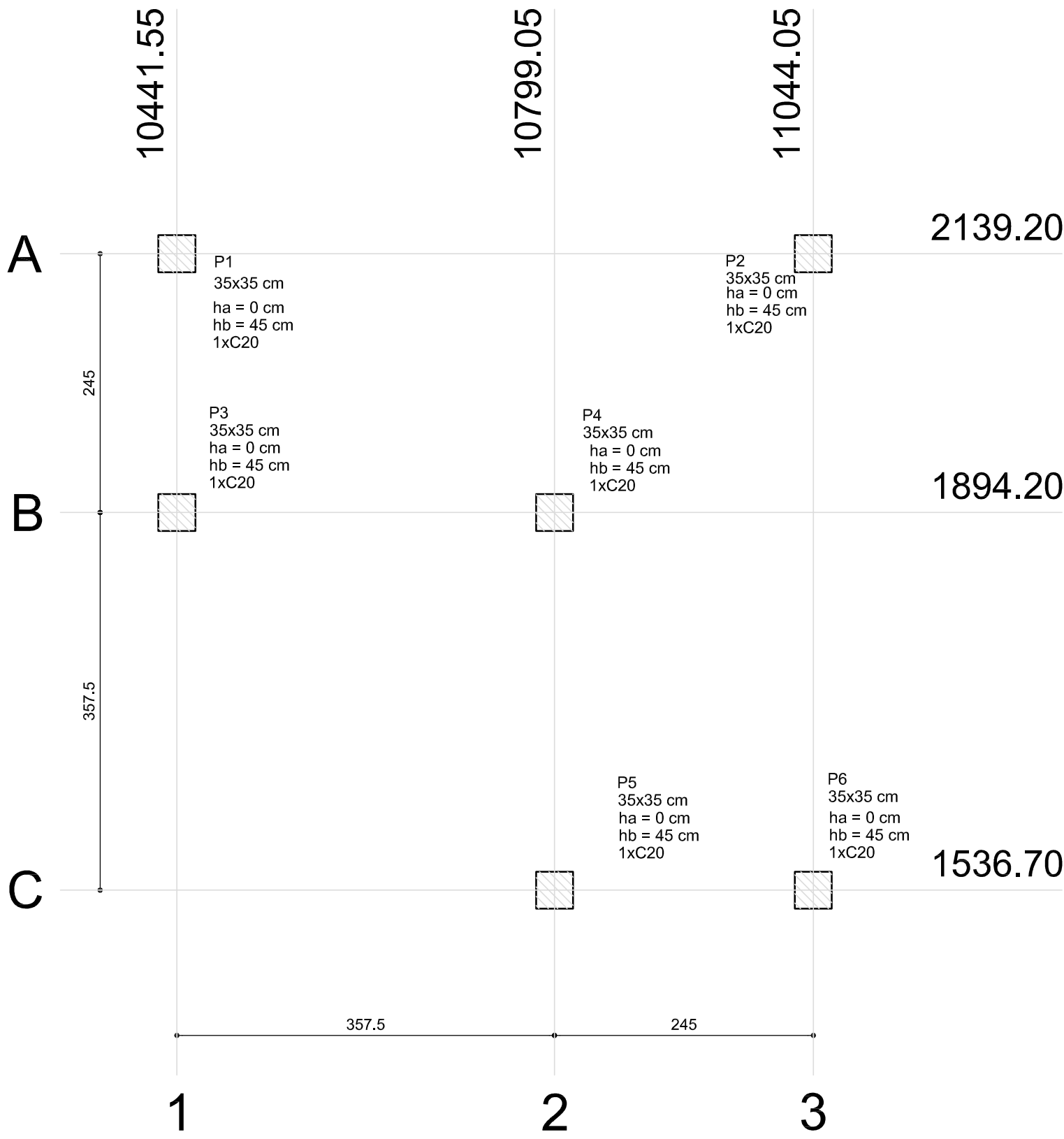
1 PLANTA DE LOCAÇÃO ESCALA 1/50
