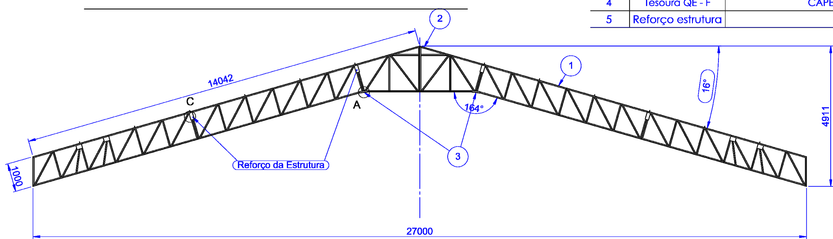
2 PÓRTICO DAS EXTREMIDADES PÓRTICO QE - B SEM ESCALA
